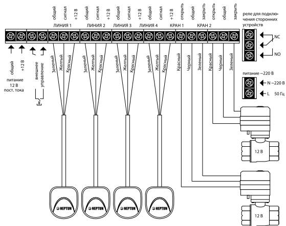
Рис. 5. Схема подключения кранов с электроприводом серии JW5000 12 VDC SS304 к модулю управления Neptun ProW
